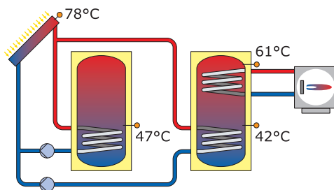
Schéma 1/3
