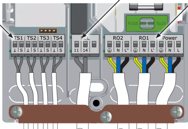
Bloque de bornes REL
