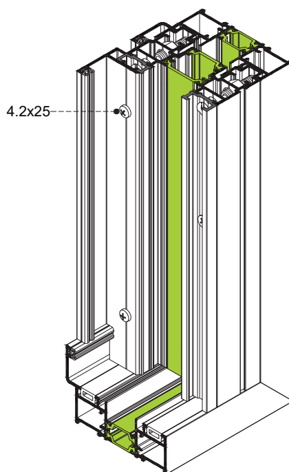
ΒΗΜΑ 4 Τοποθετούμε και βιδώνουμε το TV-77301 STEP 4 Place and screw the profile TV-77301.
