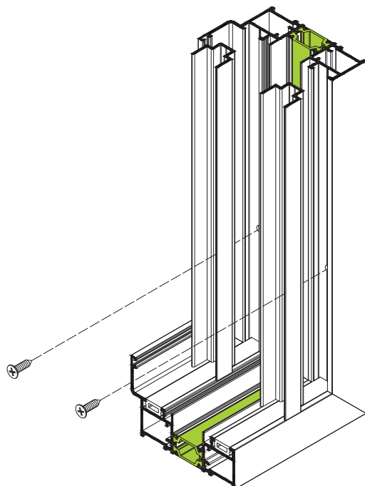
ΒΗΜΑ 1 Βιδώνουμε τα προφίλ TV-77503
