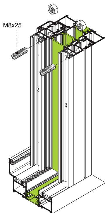
ΒΗΜΑ 3 Βιδώνουμε τις σκουλικόβιδες στα παξιμάδια STEP 3 Screw the set screws on the nuts.
