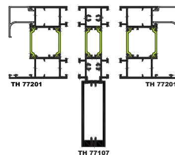
TOMH 6 SECTION 6
