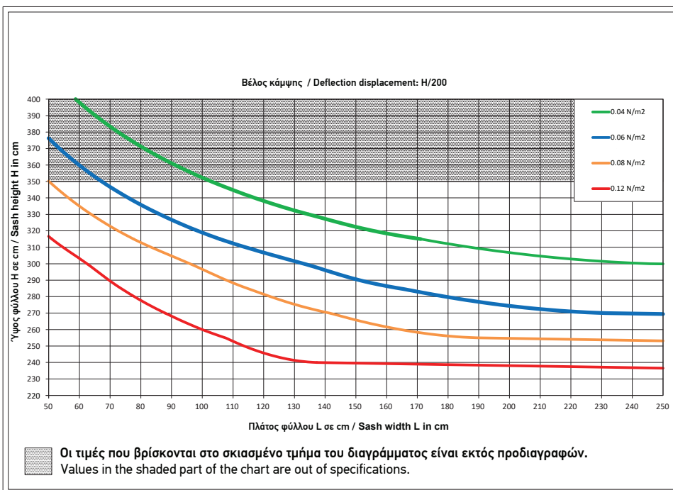
ΤΟΜΗ 4 SECTION 4
