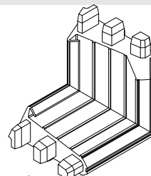
Βουλκανισμένη γωνία κεντρικού λάστιχου Vulcanized corner of central gasket
