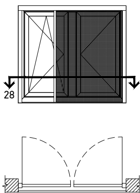
ΔΙΦΥΛΛΟ Α/Α ΜΕ ΣΗΤΑ ΠΛΙΣΣΕ DOUBLE SASH T/T WITH PLISSE INSECT SCREEN
