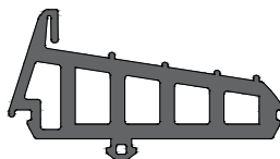
Κεντρικό Λάστιχο Κάσας Central Gasket
