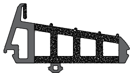
Κεντρικό Λάστιχο Κάσας Central Gasket
