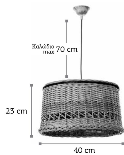
4497A 1xE27 11-42-40 Υλικό: Ρατάν
