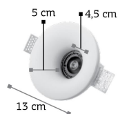
X0002 1xGU10 11-08-60 Υλικό: Γύψος
