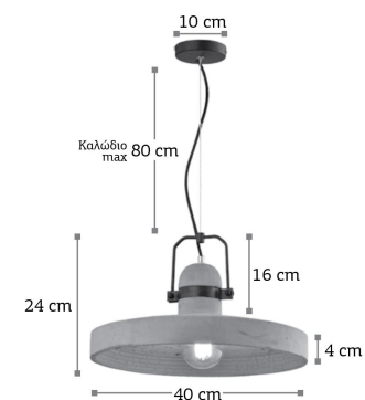
4434 1xE27 11-46-60 Υλικό: Μέταλλο-Τσιμέντο
