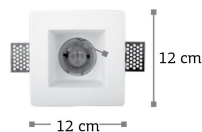
X0001 1xGU10 11-09-90 Υλικό: Γύψος
