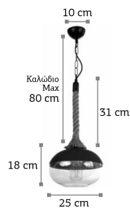
4412 1xE27 11-42-50 Υλικό: Γυαλί - Σχοινί
